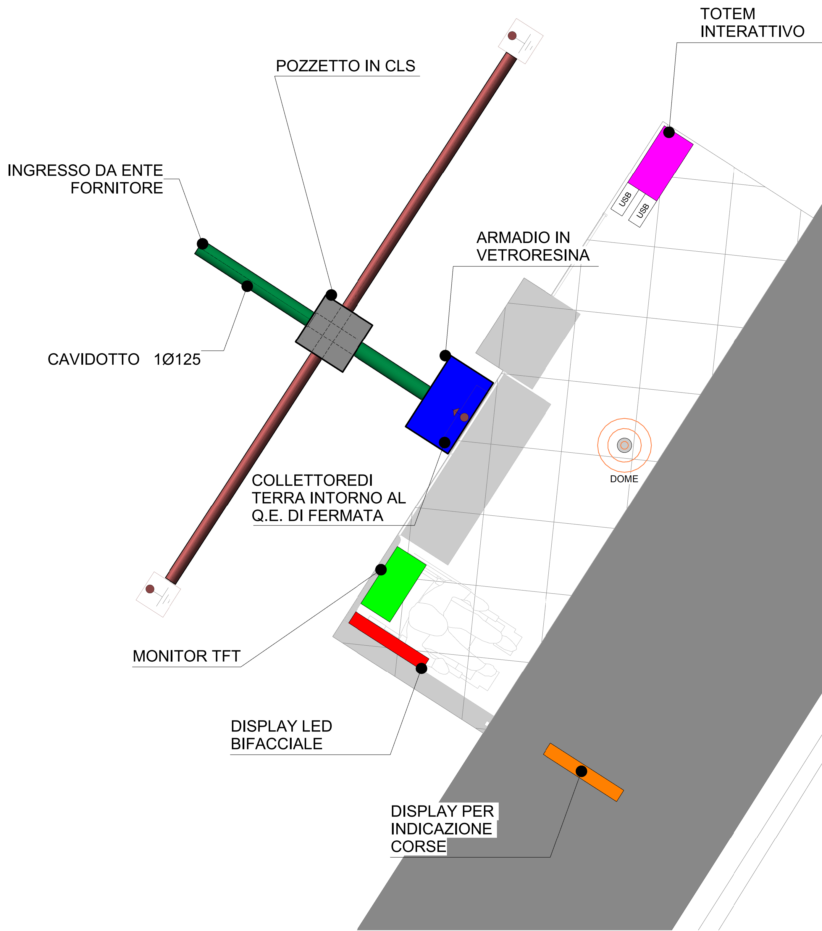
Pensilina TIPO A SCALA 1 : 20
